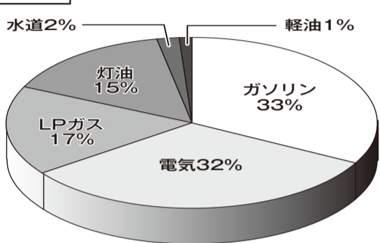
グラフ2 排出原因別二酸化炭素（CO 2 ）排出割合
