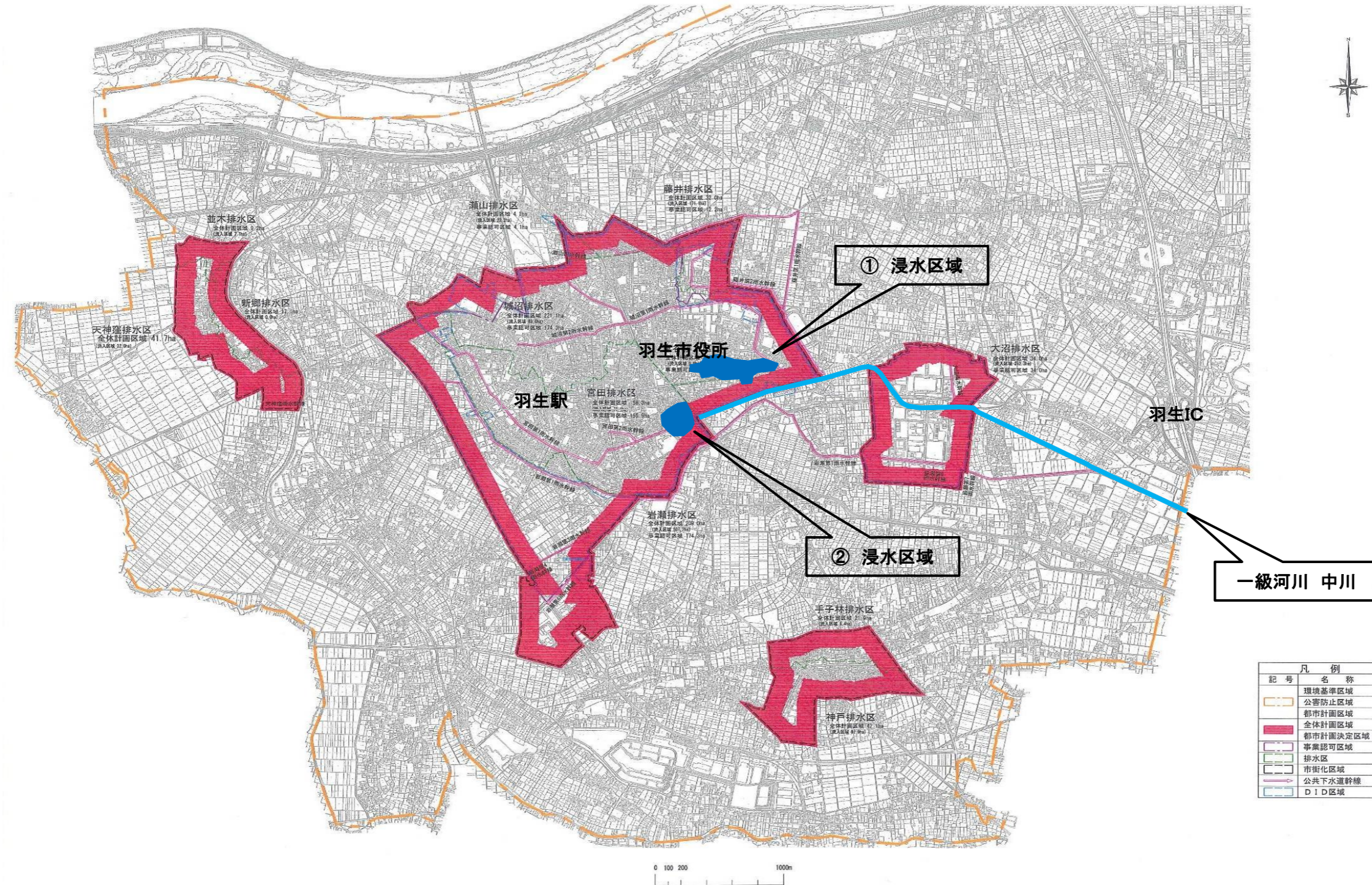
羽生公共下水道計画一般図（雨水）
