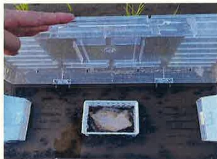
スクミリンゴガイの大量捕獲用箱型トラップ (大栄工業株式会社ウェブサイトより(引用文献リストを参照))
